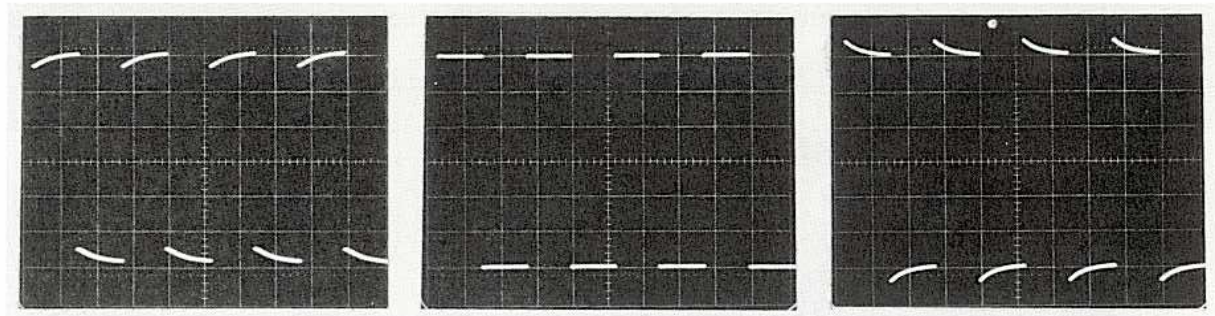
Abb. 7. Überkompensation (Einstellung C2)
